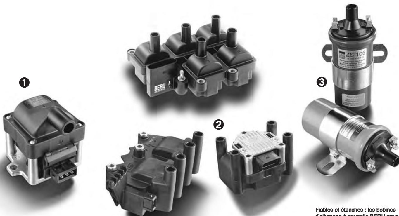
Bobines d'allumage blocs BERU pour les modèles de véhicule courants de BMW, Fiat, Renault et VW.
