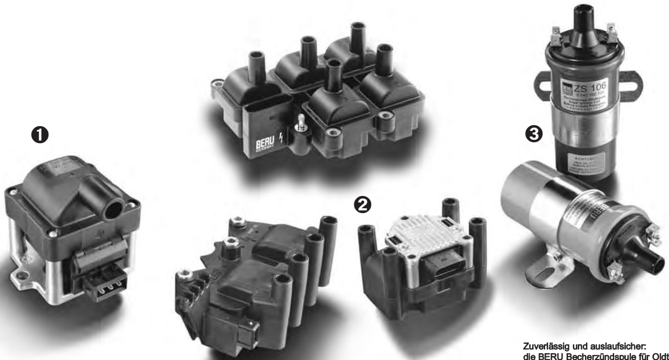
BERU Blockzündspulen für gängige Fahrzeugmodelle von BMW, Fiat, Renault und VW.
