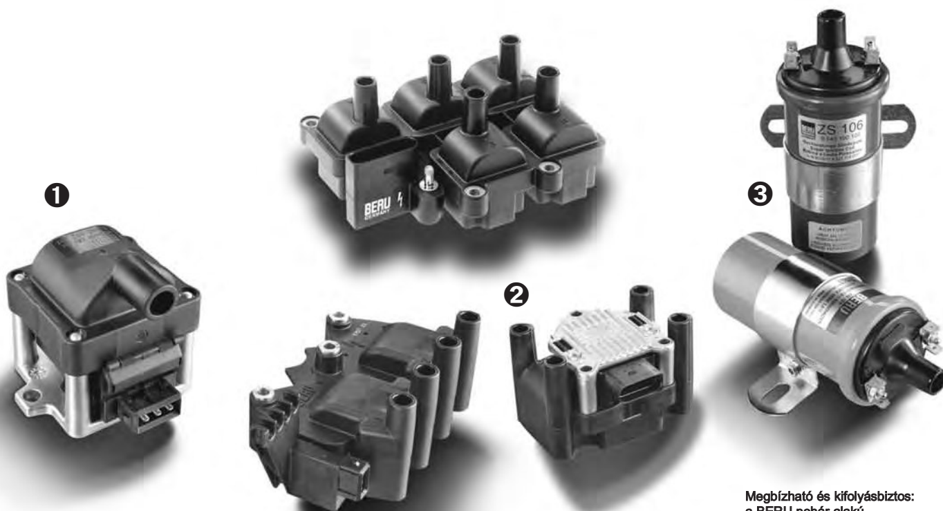
BERU tömb gyújtótekercecsek a BMW, Fiat, Renault és a VW közkedvelt gépjárműmodelljeihez.
