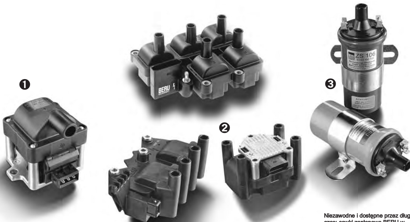
Blokowe cewki zapłonowe BERU do popularnych modeli pojazdów marki BMW, Fiat, Renault i VW.
